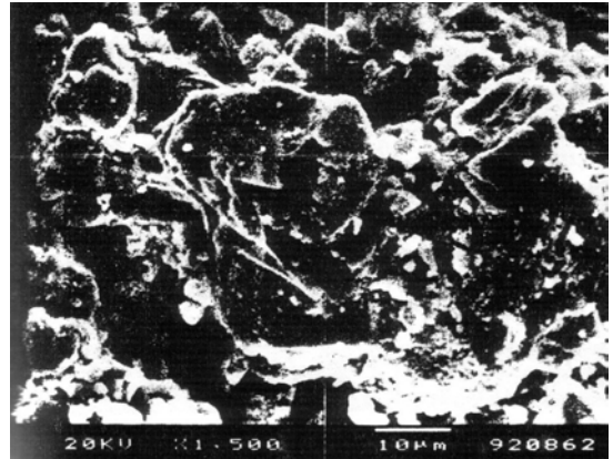
NiSO 4
