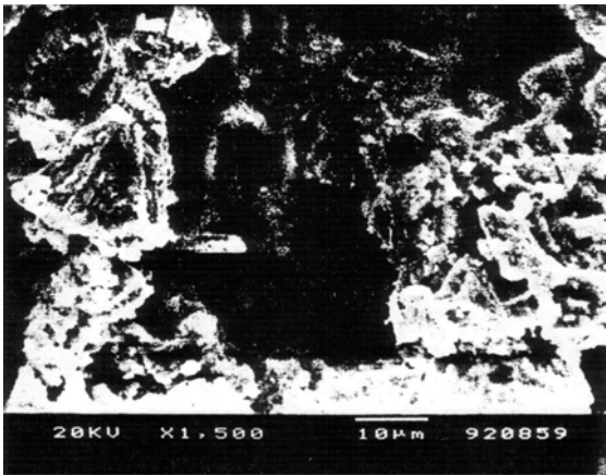
NiSO 4 (*)
