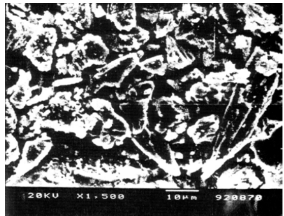
CuSO 4
