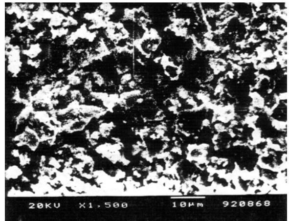
CuSO 4
