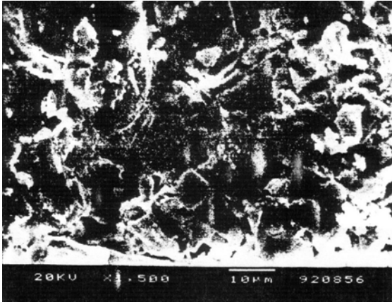
NiSO 4 (*)
