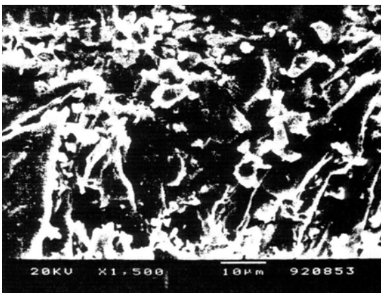
CuSO 4 (*)
